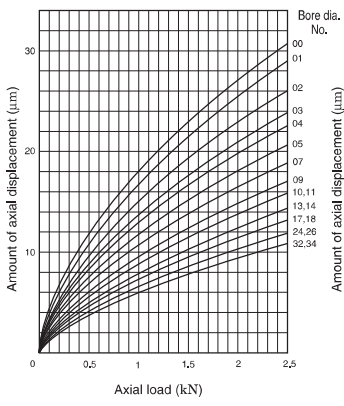
(4) 7000 (contact angle 30°)
