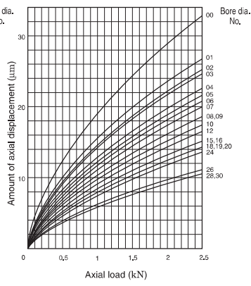
(5) 7200 (contact angle 30°)
